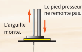
Le tissu est maintenu. Avec DCP*
