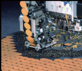
Dispositif IV pose paillettes
