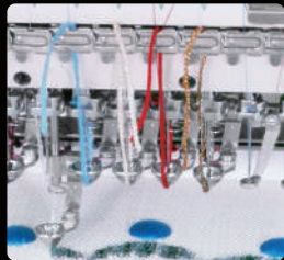
Dispositif pose cordons multiples
